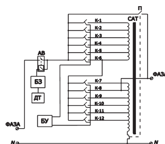
Структурная схема стабилизатора (36 ступеней)
