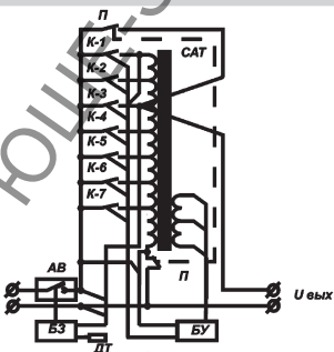
Структурная схема стабилизатора (7 ступеней)
